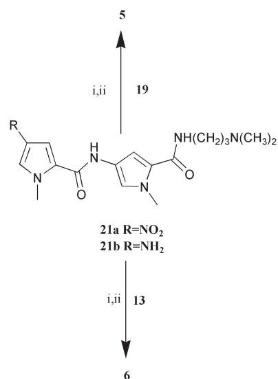
Scheme 3 i) Pd/C/H 2 ; ii) HBTU/NMM/DMF.
