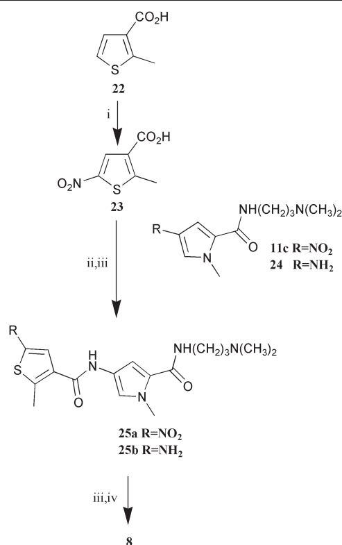
Scheme 4 i) HNO 3 /H 2 SO 4 ; ii) 23 , SOCl 2 ; iii) 11c , Pd/C/H 2 ; iv) 19 , SOCl 2 .
